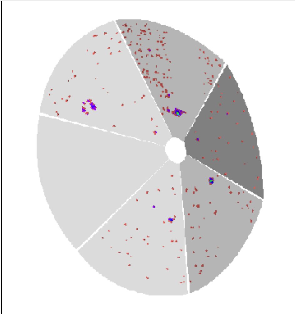
Abbildung 4.1: Ein Einzelereignis des RICH, in dem sich ein Ring befindet. Der Sektor ohne Signal ist der einzige noch nicht mit Elektronik bestückte Sektor. In diesem Ereignis war kein Magnetfeld eingeschaltet.
