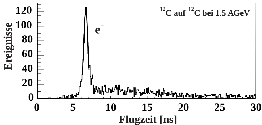
Abbildung 4.7: Alle Einträge aus Abbildung 4.6, die mit einem Leptonenkandidaten des RICH korreliert sind [Thú00].
