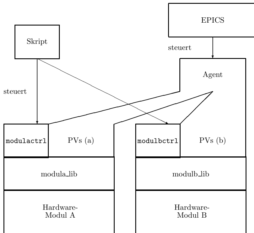
Abbildung 3.6: Gemeinsame Nutzung der Hardwarebibliotheken durch ctrl -Programme und Agenten.
