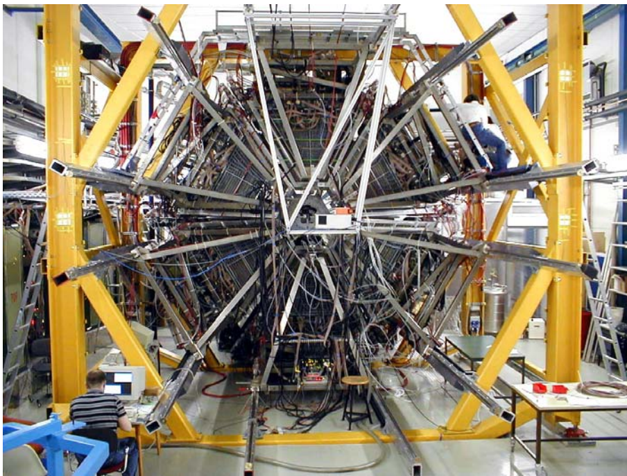
Abbildung 1.2: HADES im November 2000.
