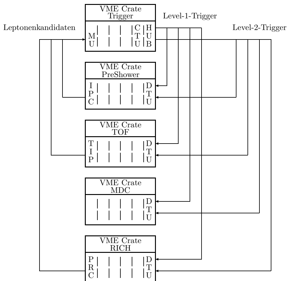
Abbildung 2.4: Aufbau des mehrstufigen HADES Triggersystems; IPC, TIP und PRC sind die Bildverarbeitungseinheiten der verschiedenen Detektoren.
