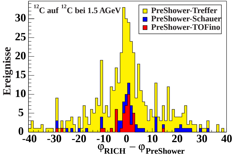
Abbildung 4.2: Die diesem Spektrum zugrundeliegenden Daten wurden ohne Magnetfeld aufgenommen. Gezeigt sind Ereignisse mit Signalen, die in beiden Detektoren jeweils den gleichen Polarwinkel haben [Fab00].
