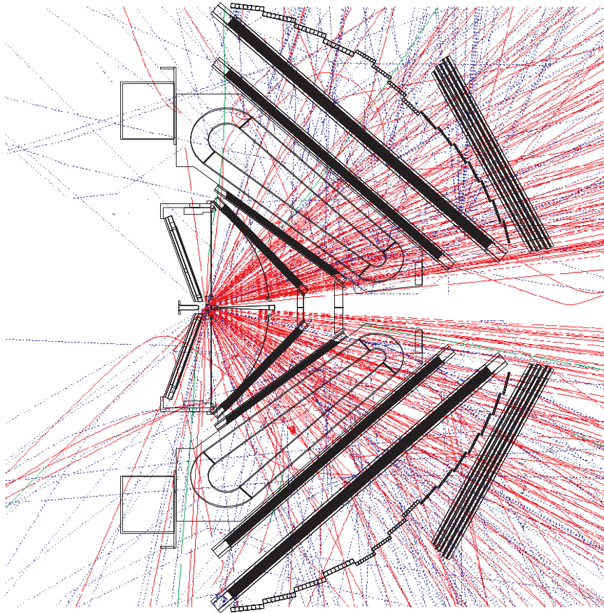
Abbildung 2.2: Bei einer zentralen Kollision zweier Goldkerne mit einer Schwerpunktsenergie von 1 AGeV werden etwa 200 geladene Teilchen erzeugt.
