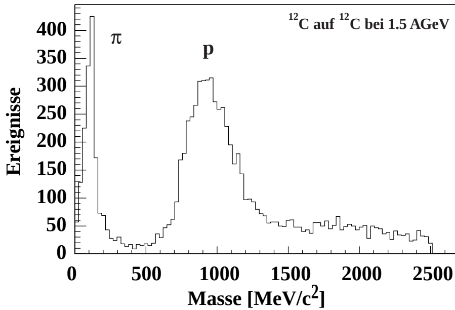
Abbildung 4.5: Spektrum der Gesamtenergie, das \pi^+ und \pi^- von Protonen separiert [Sán00].
