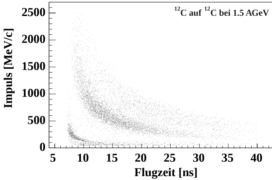
Abbildung 4.4: Impulse gegen die Flugzeit aufgetragen [Sán00].
