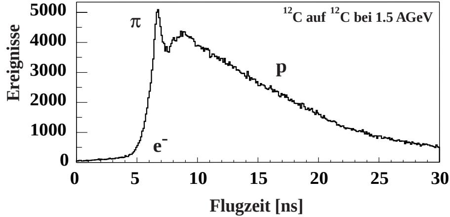
Abbildung 4.6: Ein Flugzeitspektrum von HADES-TOF [Thú00].
