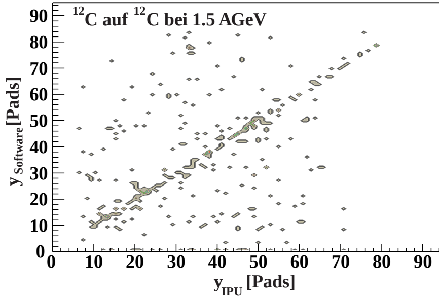
Abbildung 4.8: Radiale Ortsverteilung von Ringmittelpunkten, die „online“ in der IPU gefunden wurden, gegen die Mittelpunkte, die nachträglich mit der Analysesoftware aus allen Daten herausgefiltert wurden [Küh00]. Die Korrelation ist eindeutig zu erkennen.
