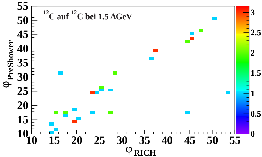
Abbildung 4.3: Hier sind für alle „PreShower-TOFino“ Ereignisse aus Abbildung 4.2 die Polarwinkel \varphi_{RICH} und \varphi_{PreShower} gegeneinander aufgetragen [Kid00].
