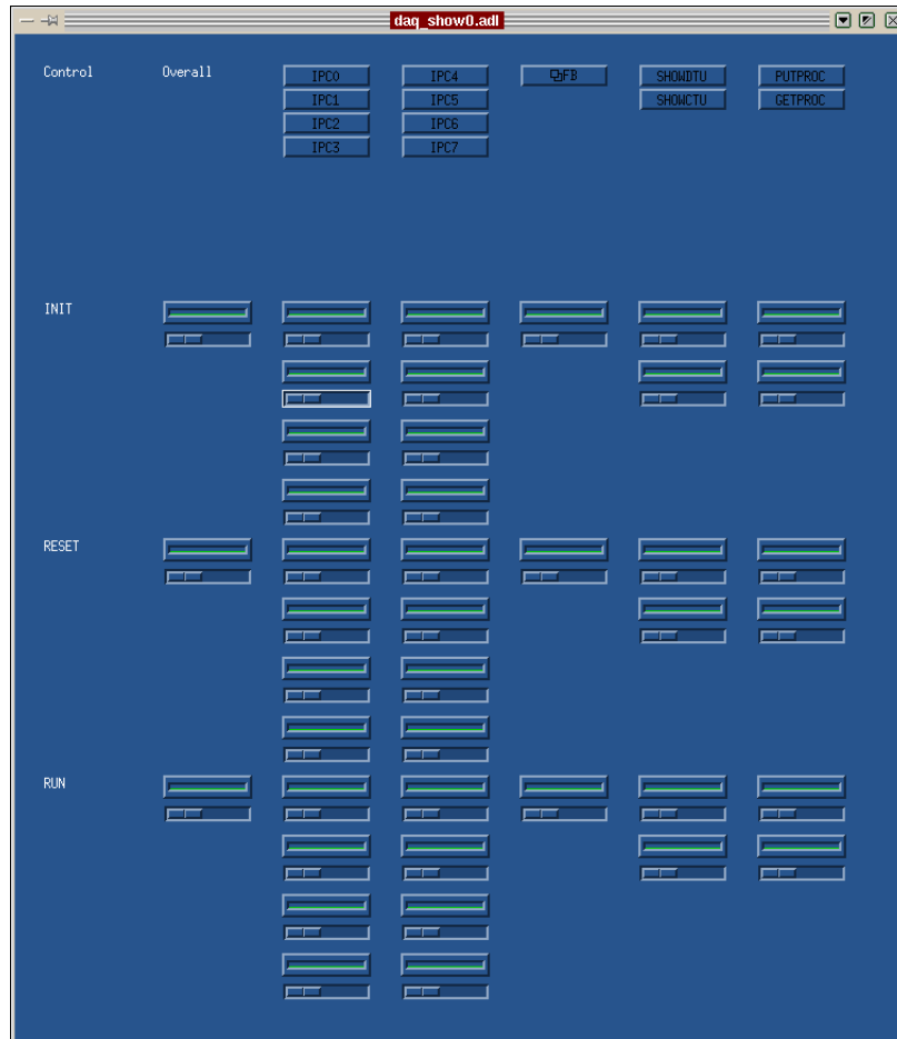
Abbildung 3.9: Die dynamisch erzeugte, graphische Benutzeroberfläche; im oberen Bereich der Maske sind Bestandteile des kontrollierten VME-Crates aufgelistet. In diesem Fall ist der Inhalt des PreShower-Auslese-Crates dargestellt. Die ersten beiden Spalten enthalten die Bildverarbeitungseinheiten, dann folgt ein „Fanout Board“, die DTU und die CTU und ganz rechts die beiden Datenaufnahmeprozesse. Unter den Knöpfen, die zu Detailinformationen über die Module führen, finden sich Statusanzeigen und Kontrollelemente für die jeweiligen „INIT“- „RESET“- und „RUN“-PVs. Links davon finden sich die entsprechenden Elemente für das gesamte VME-Crate.
