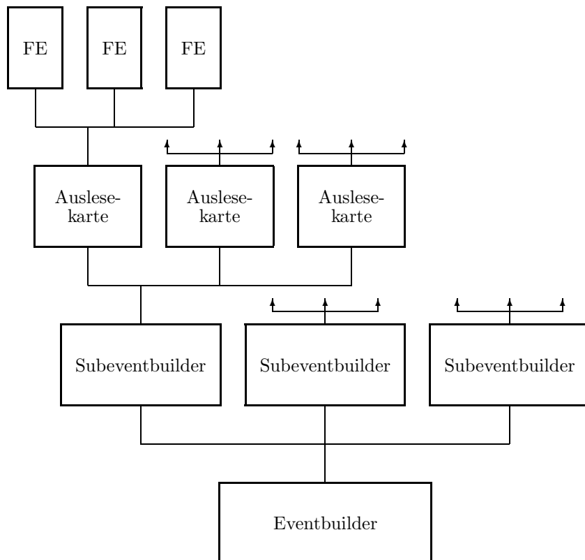
Abbildung 2.7: Überblick über die hierarchische Struktur der Datenaufnahme.
