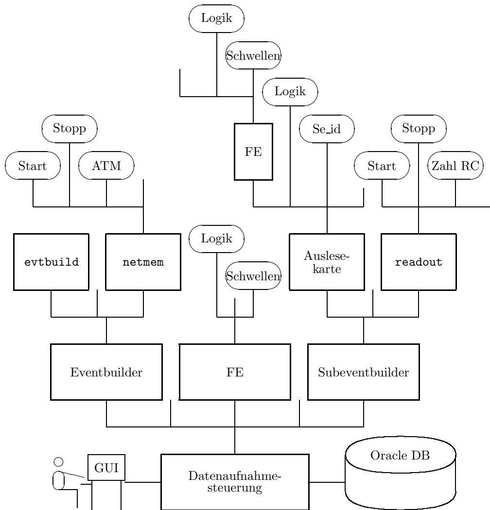
Abbildung 3.1: Die Struktur der Datenaufnahme aus Sicht der Datenaufnahme-steuerung; nur ein kleiner Teil der bereitzustellenden Funktionalität ist in den Blättern des Baumes dargestellt.
