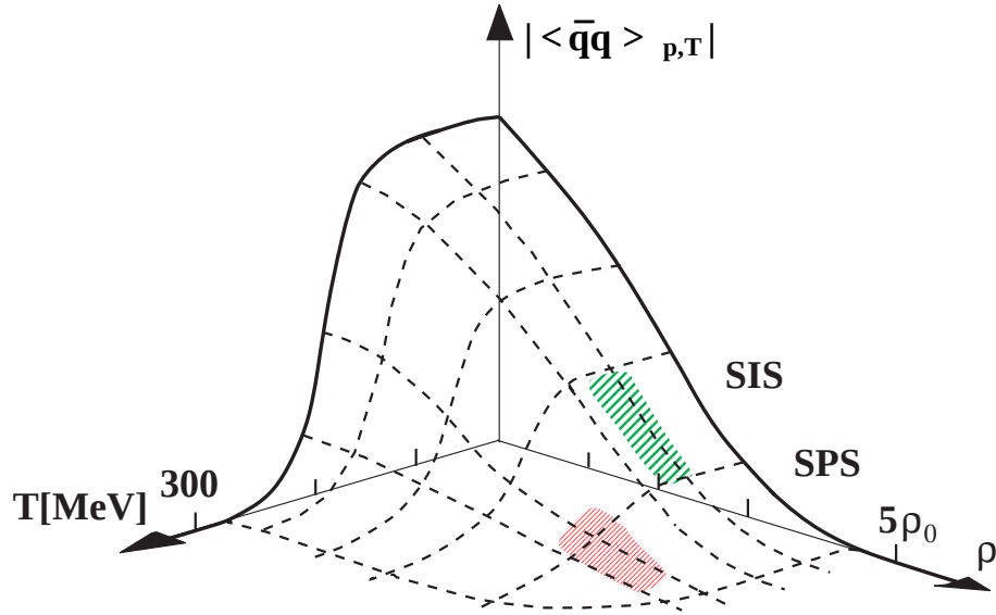
Abbildung 1.1: Restauration der chiralen Symmetrie bei hohen Temperaturen und Dichten nach Weise [Wei94]. Die Wahrscheinlichkeitsdichte des Quark-Antiquark-Kondensats nimmt ab, was mit einer Verringerung der Masse von leichten Vektormesonen einhergeht.
