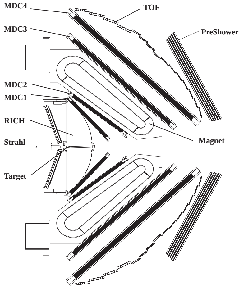
Abbildung 2.1: Schnitt durch das HADES Detektorsystem.
