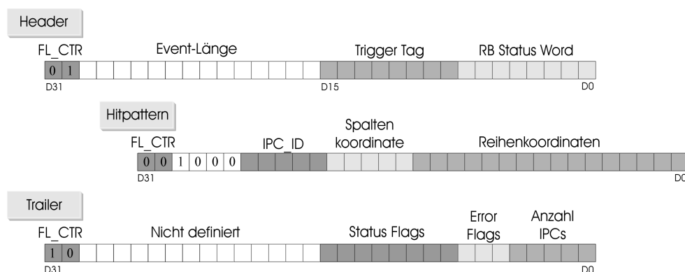
Abbildung 5.21: Struktur der Hitpattern-Subevents, die vom Link Module zur Matching Unit übertragen werden.
