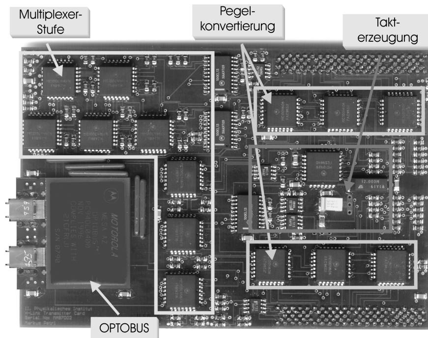
Abbildung 6.4: Das als Aufsteckkarte (138 mm x 92 mm) realisierte H-Link-System (Transmitter). Funktionale Einheiten sind durch Rahmen zusammengefaßt.
