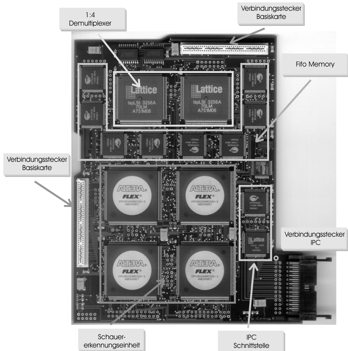
Abbildung 5.18: Die Erweiterungskarte. Die in den vorhergehenden Kapiteln beschriebenen funktionalen Einheiten sind durch Rahmen zusammengefaßt.
