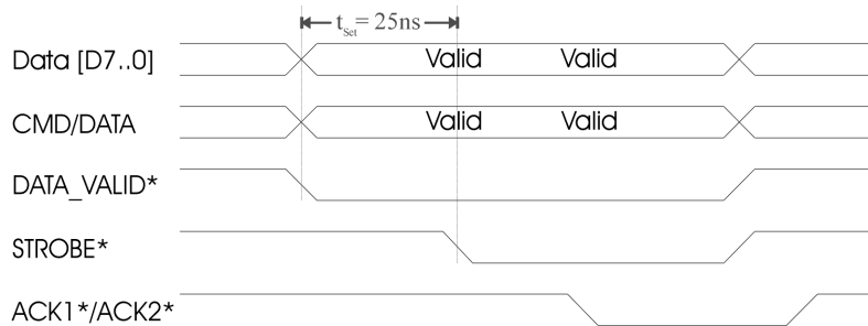
Abbildung 5.2: Timing Diagramm für die Übertragung der Auslesebefehle und Testdaten zwischen Fanout Board und Front-End Elektronik.
