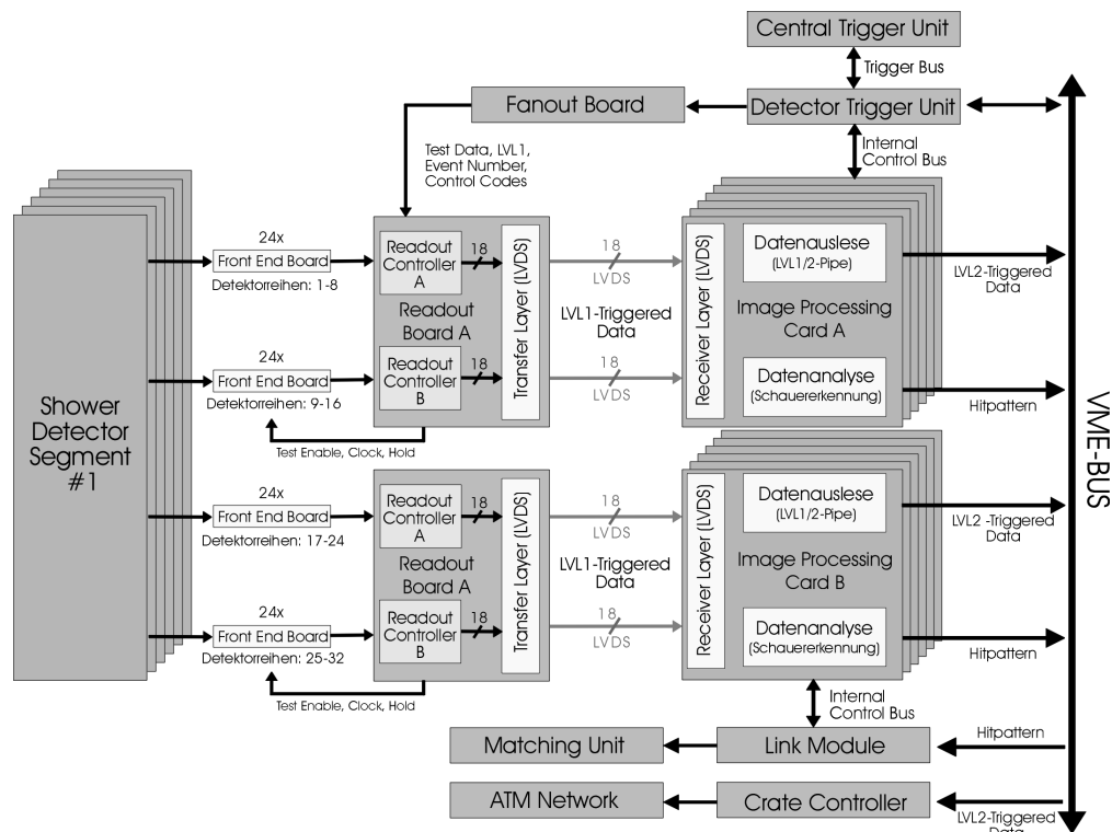
Abbildung 5.1: Schematische Darstellung des Trigger- und Auslesesystems für den HADES-Schauerdetektor. Nach dem Erhalt eines LVL1-Triggers startet die lokale Detector Trigger Unit die Detektorauslese sowie die erste Stufe der Datenverarbeitung durch die Front-End-Elektronik. Die in diesem Schritt erzeugten digitalen Ladungswerte der einzelnen Kathodenfelder werden von den Readout Boards zu den Image Processing Cards übertragen, wo eine Zwischenspeicherung in der LVL1/LVL2-Pipe sowie die eigentliche Datenanalyse stattfindet. Eine Weiterleitung der Analyseergebnisse an die Matching Unit erfolgt durch das Link Module. Die von der Matching Unit bestimmte LVL2-Triggerentscheidung wird via CTU-DTU an die IPCs verteilt, die in Abhängigkeit dieser Entscheidung die entsprechenden Daten der LVL1-Pipe verarbeiten.
