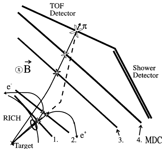
Abbildung 3.3: Beispiel für ein falsch im LVL2-Trigger identifiziertes Lepton. Ein Elektron/Positron Paar aus einem Untergrundprozeß erzeugt einen Ring im RICH, der mit einem hochenergetischen Pion kombiniert wird. Die gestrichelte Linie zeigt die vom LVL3-Trigger geforderte Teilchenspur in den MDC-Ebenen 1 bis 4.
