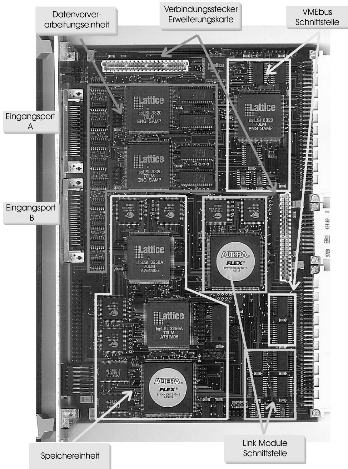
Abbildung 5.17: Die im 6U VME-Standard realisierte Basiskarte. Die in den vorhergehenden Kapiteln beschriebenen funktionalen Einheiten sind durch Rahmen in unterschiedlichen Graustufen zusammengefaßt.
