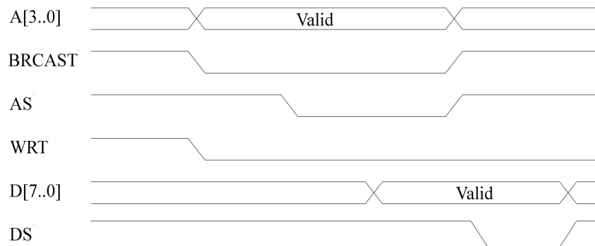
Abbildung 5.13: Relative Timing-Diagramm für einen Broadcast-Write-Zyklus, der zur Übertragung der LVL2-Triggerentscheidung zwischen der DTU und den 12 IPCs verwendet wird. Das Trigger-Tag und der Trigger-Code werden in zwei aufeinanderfolgenden Zyklen über die Datenleitungen übertragen.
