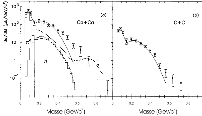
Abbildung 1.8: Mit dem DLS gemessene Dileptonenspektren für die Reaktionen \text{Ca}+\text{Ca} bzw. \text{C}+\text{C} bei 1 AGeV. Die durchgezogene Kurve ist ein Fit an die Daten bei niedrigen Massen unter Berücksichtigung der bekannten Dileptonenquellen. Die gepunktete Kurve ist eine BUU-Rechnung. Die Histogramme zeigen eine Abschätzung der zu erwartenden \pi^0 - und \eta -Beiträge basierend auf TAPS-Messungen ([Ber94], [Sch94]) und einem isotropen thermischen Modell [Por97].
