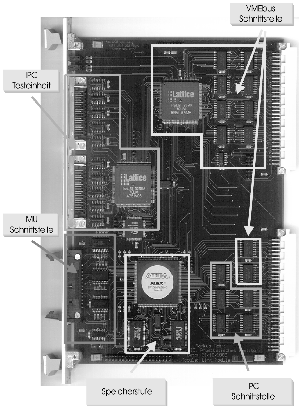
Abbildung 5.22: Das als 6U-VME-Karte realisierte Link Module. Die vorab beschriebenen funktionalen Einheiten und Schnittstellen sind durch Boxen zusammengefaßt.
